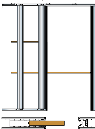
Horizontální řez jednokřídlého pouzdra
